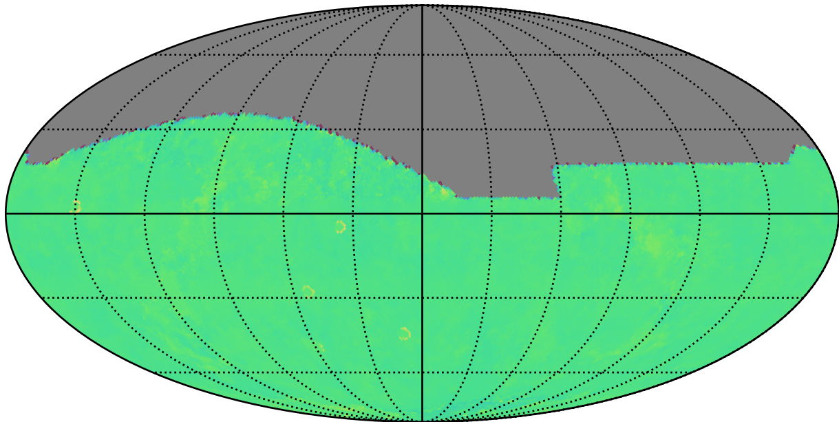
too_elab_2yr_r32_d2_ugrizy_v3.4_10yrs z: Kuiper rotTelPos
