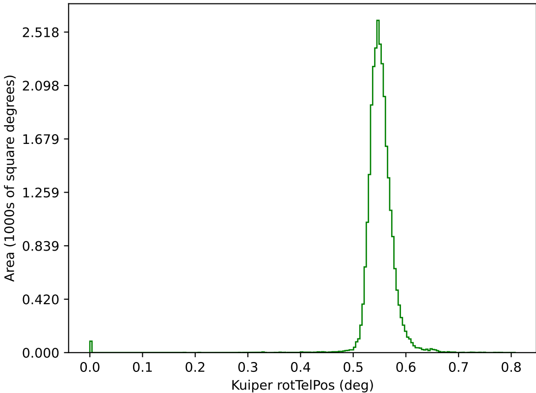
too_elab_2yr_r32_d2_ugrizy_v3.4_10yrs g: Kuiper rotTelPos
