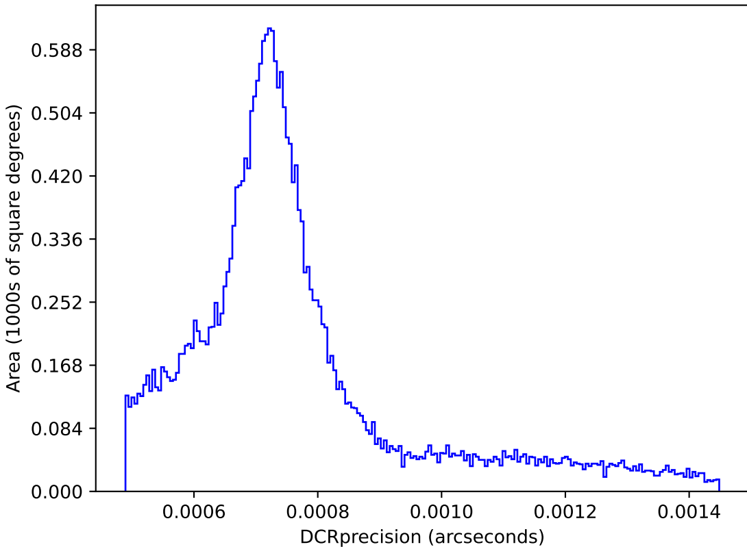
too_elab_2yr_r32_d2_ugrizy_v3.4_10yrs : DCRprecision
