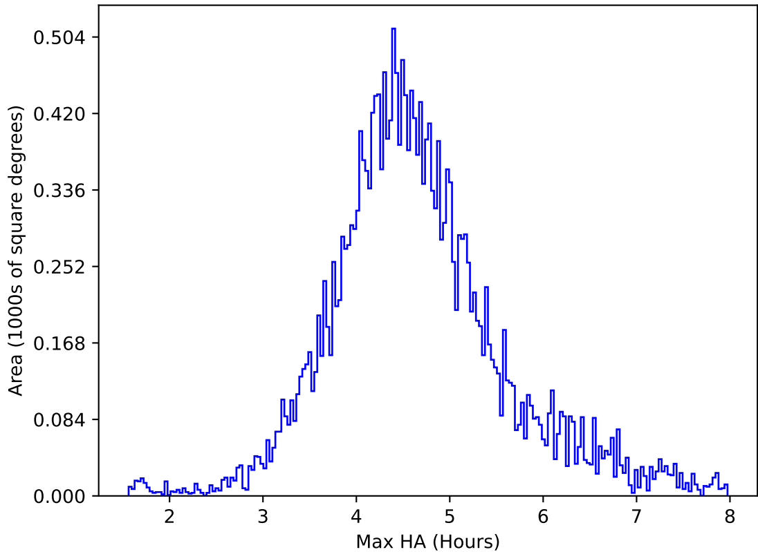
too_elab_2yr_r32_d2_ugrizy_v3.4_10yrs All sky y band: Max HA
