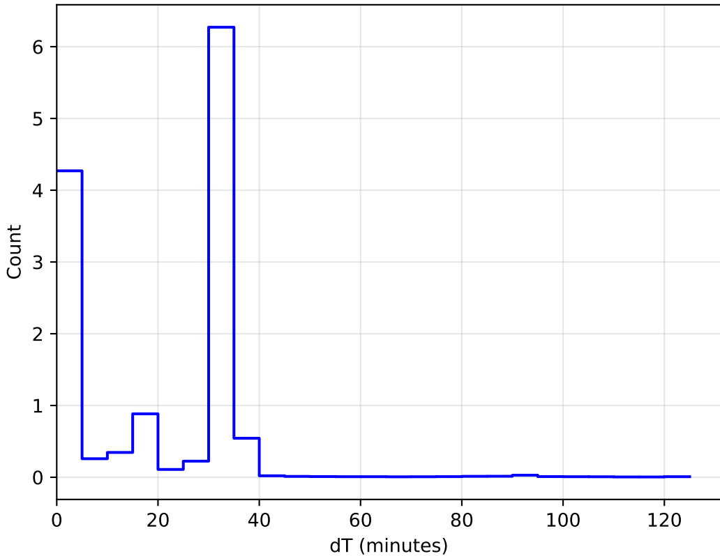
too_elab_2yr_r32_d2_ugrizy_v3.4_10yrs All sky: DeltaT Histogram 1e6
