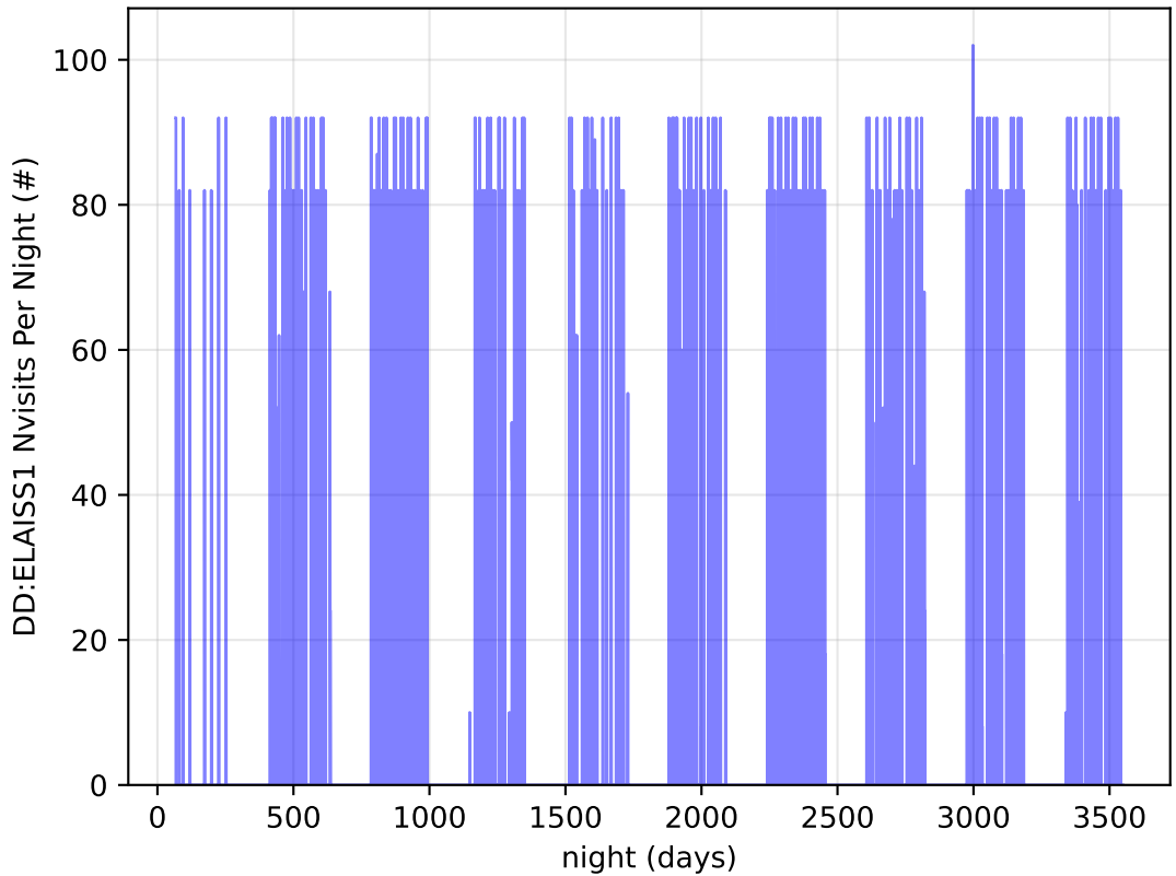
too_elab_2yr_r32_d2_ugrizy_v3.4_10yrs all bands: DD:ELAISS1 Nvisits Per Night
