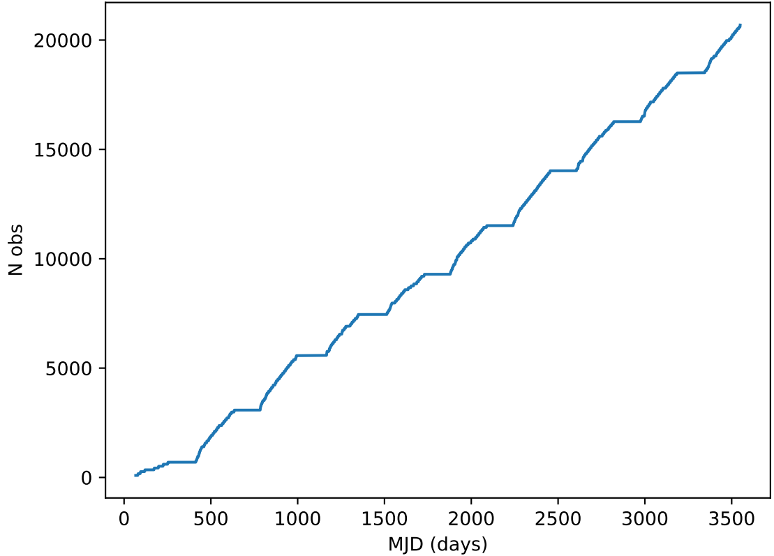
too_elab_2yr_r32_d2_ugrizy_v3.4_10yrs all bands: DD:ELAISS1 Cumulative NVisits
