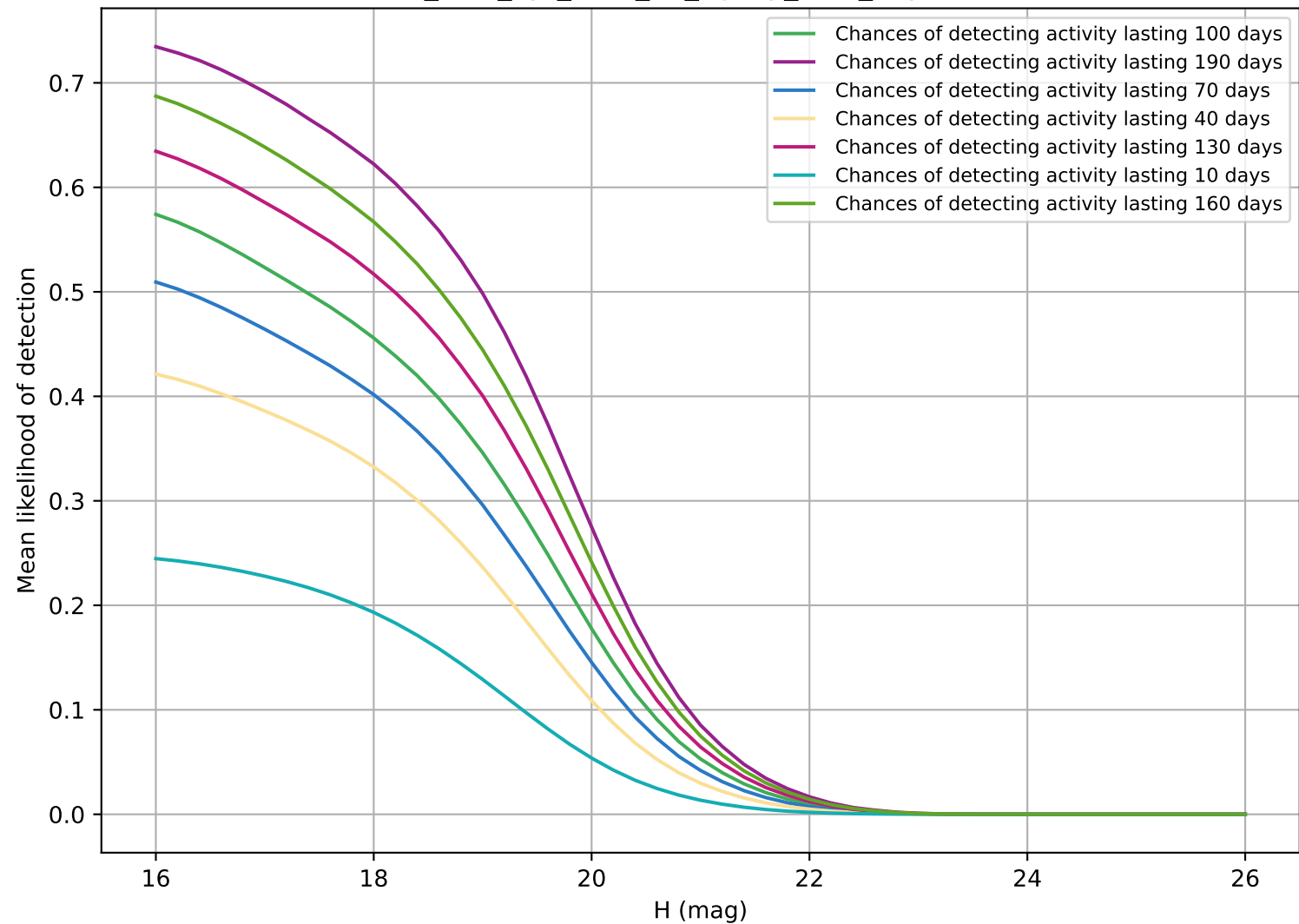
too_elab_2yr_r128_d3_ugrizy_v3.4_10yrs MBA
