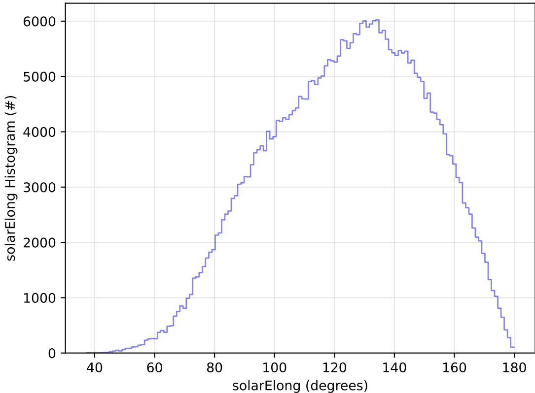
too_elab_2yr_r128_d3_ugrizy_v3.4_10yrs All sky y band: solarElong Histogram
