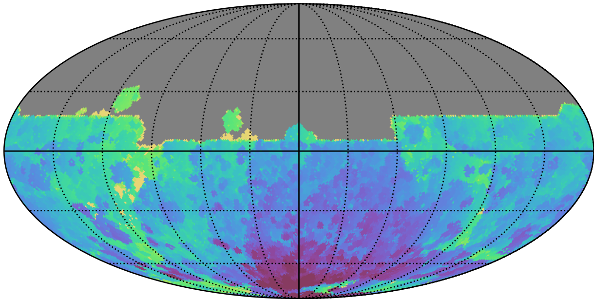
too_elab_2yr_r128_d3_ugrizy_v3.4_10yrs All sky y band: Min HA
