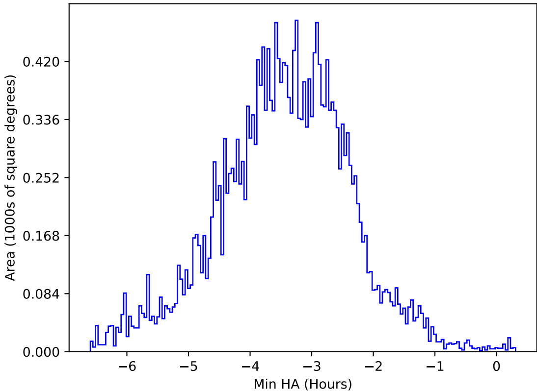
too_elab_2yr_r128_d3_ugrizy_v3.4_10yrs All sky y band: Min HA
