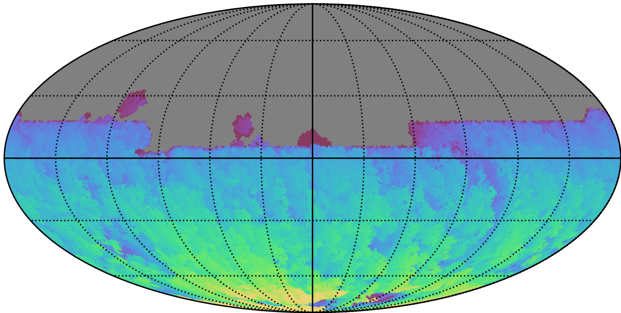
too_elab_2yr_r128_d3_ugrizy_v3.4_10yrs All sky y band: Max HA
