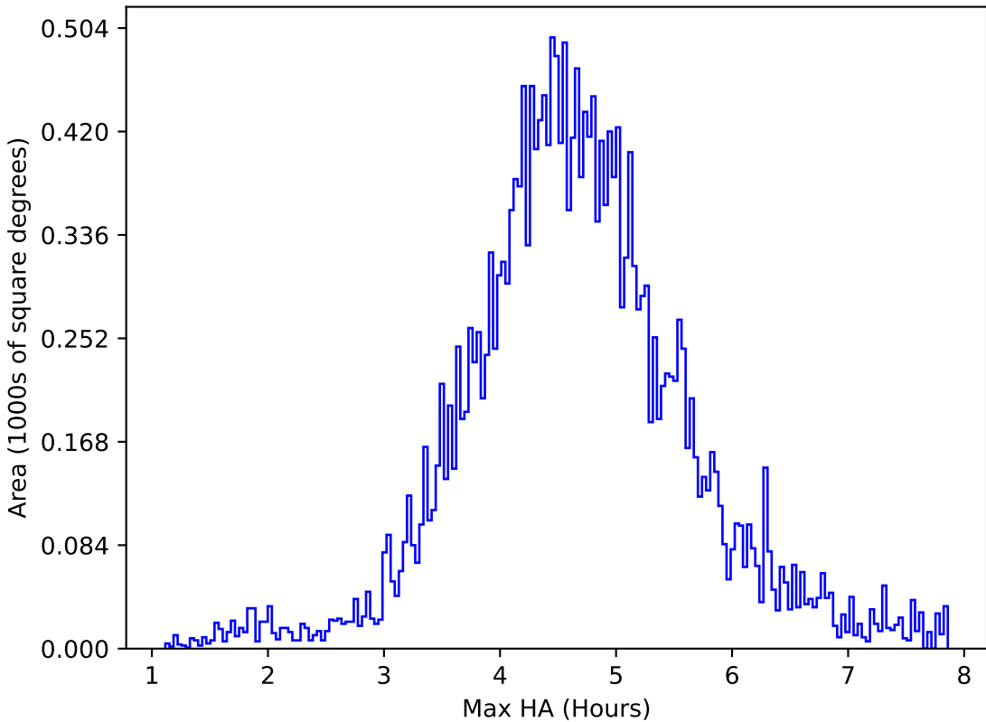
too_elab_2yr_r128_d3_ugrizy_v3.4_10yrs All sky y band: Max HA
