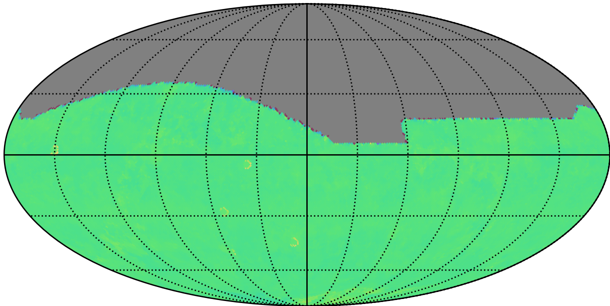
too_elab_2yr_r128_d2_ugrizy_v3.4_10yrs i: Kuiper rotTelPos
