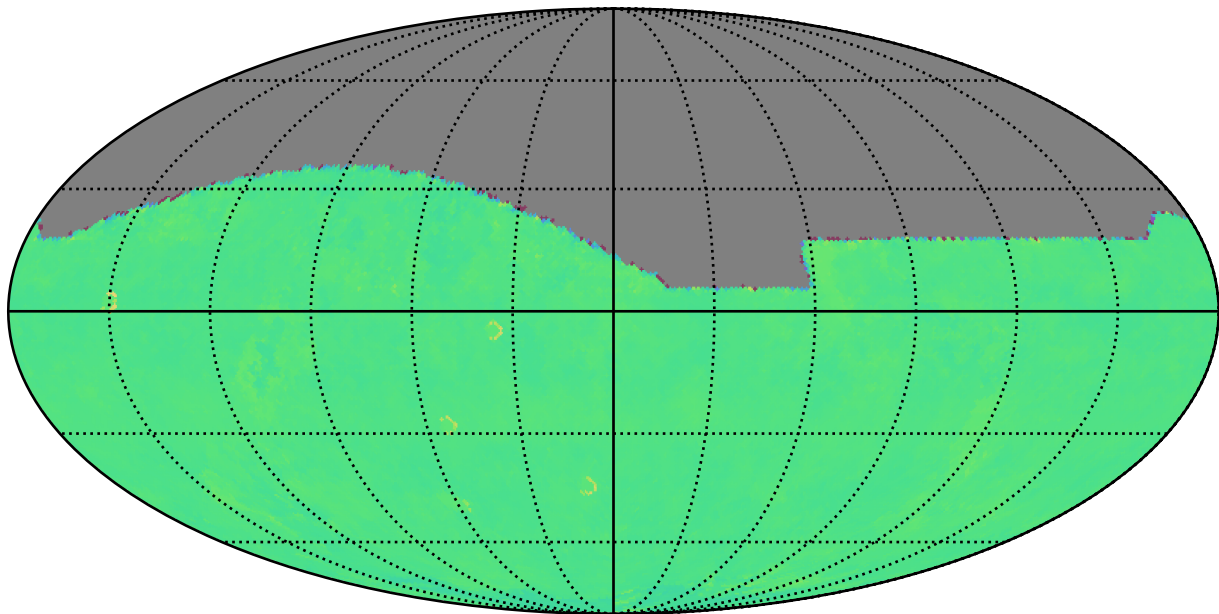
too_combined_s2.0_v3.4_10yrs i: Kuiper rotTelPos
