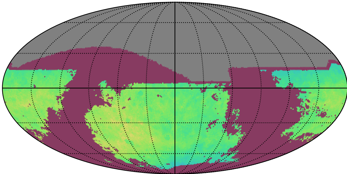
too_combined_s1.5_v3.4_10yrs i: NgalScale
