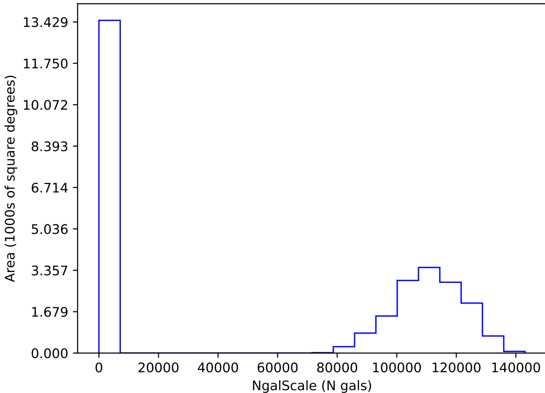
too_combined_s1.5_v3.4_10yrs i: NgalScale
