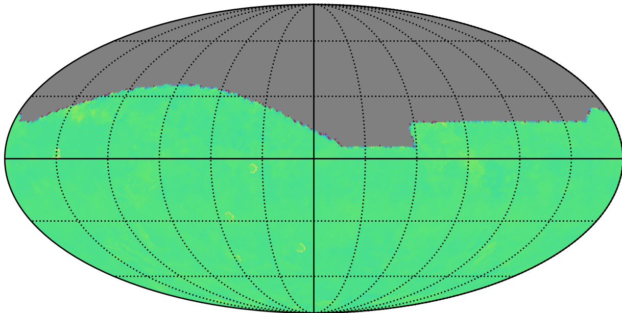
too_combined_s1.5_v3.4_10yrs i: Kuiper rotTelPos
