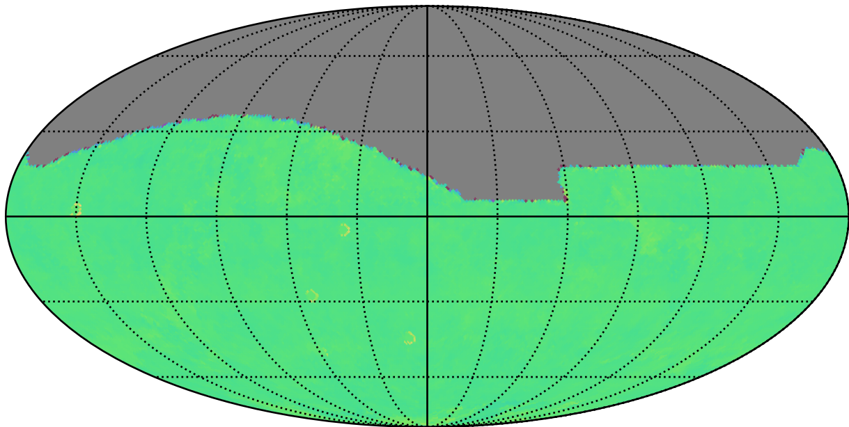
too_combined_s1.0_v3.4_10yrs i: Kuiper rotTelPos
