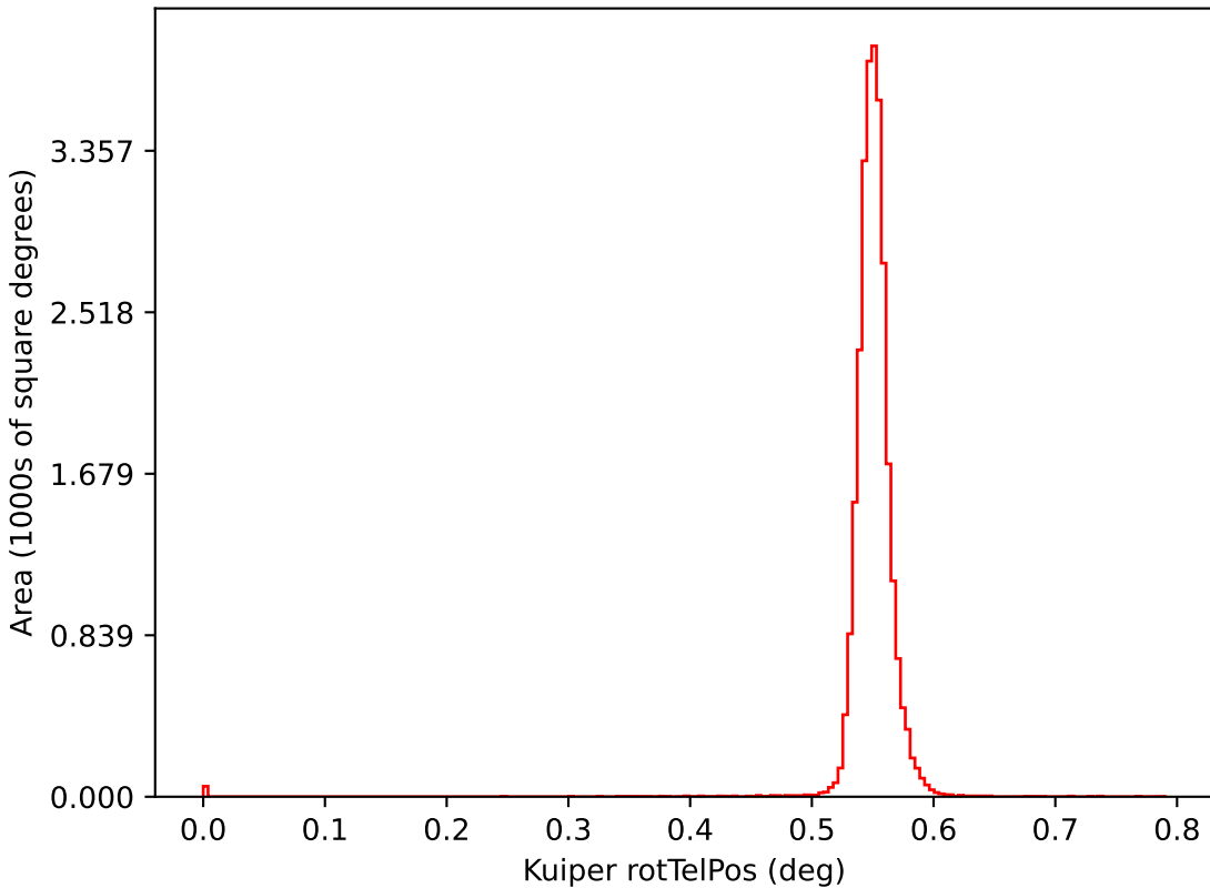
too_combined_s1.0_v3.4_10yrs i: Kuiper rotTelPos
