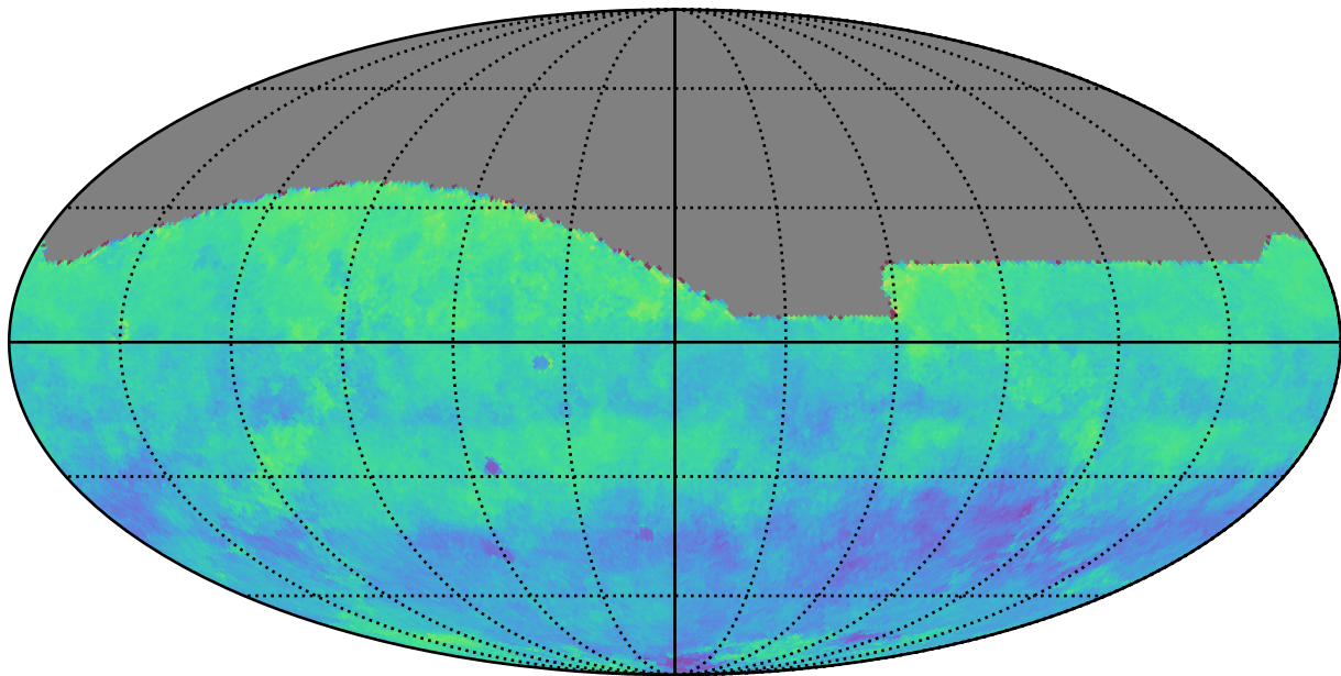
too_combined_s1.0_v3.4_10yrs i: Kuiper rotSkyPos
