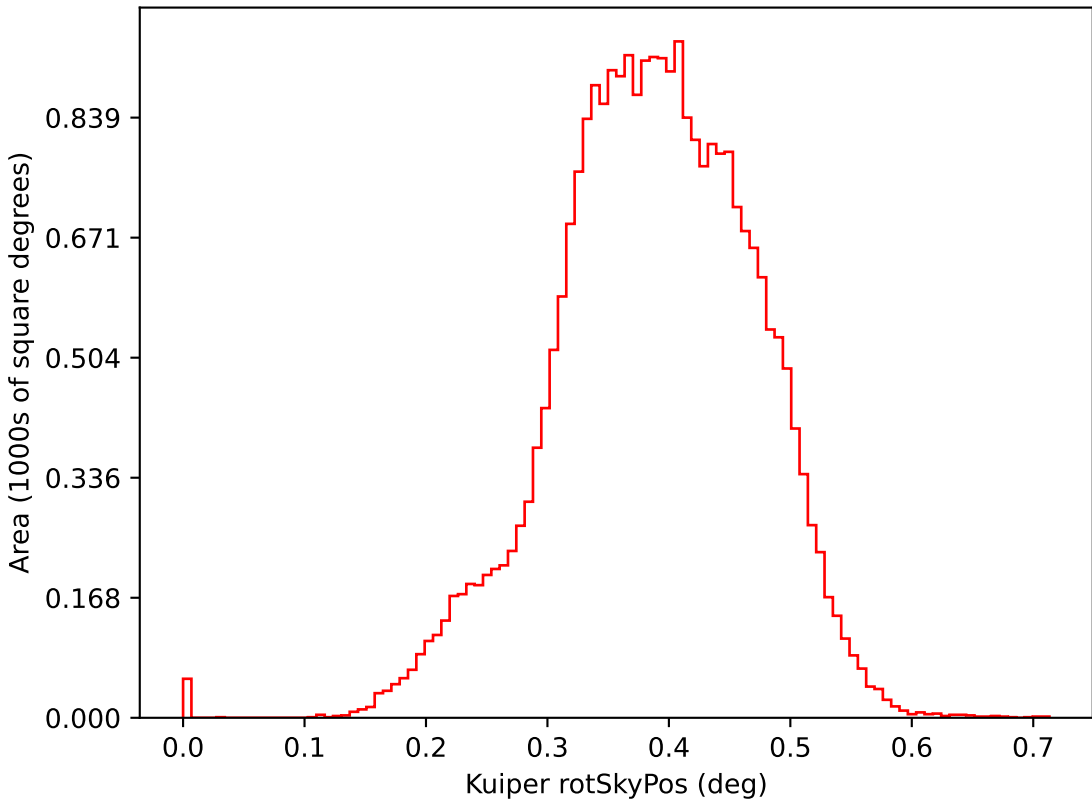
too_combined_s1.0_v3.4_10yrs i: Kuiper rotSkyPos
