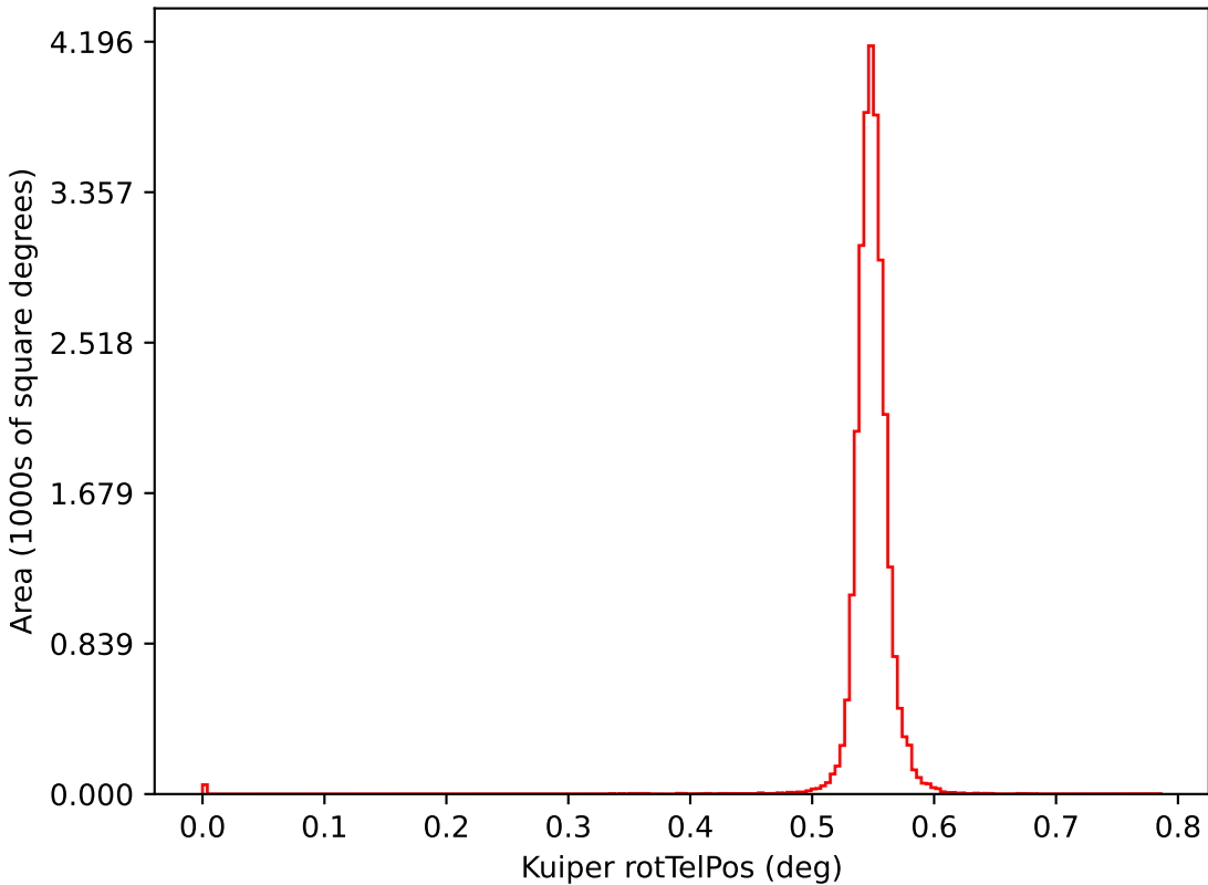
too_combined_s0.8_v3.4_10yrs i: Kuiper rotTelPos
