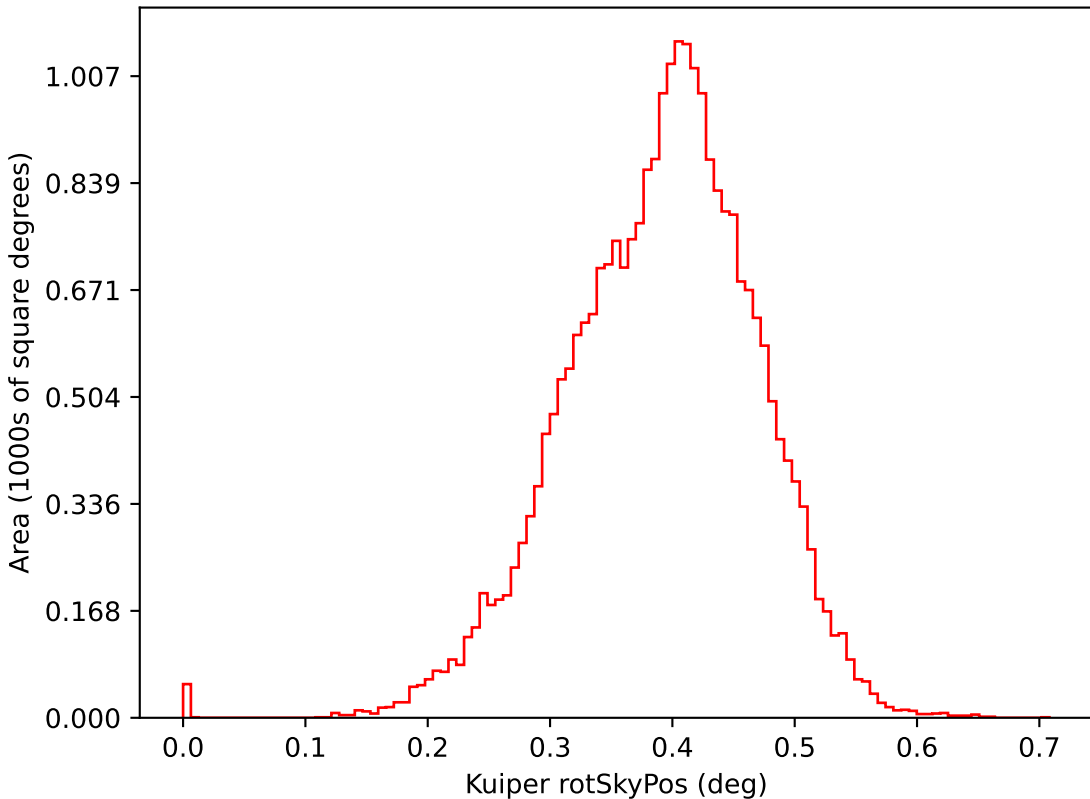
too_combined_s0.8_v3.4_10yrs i: Kuiper rotSkyPos
