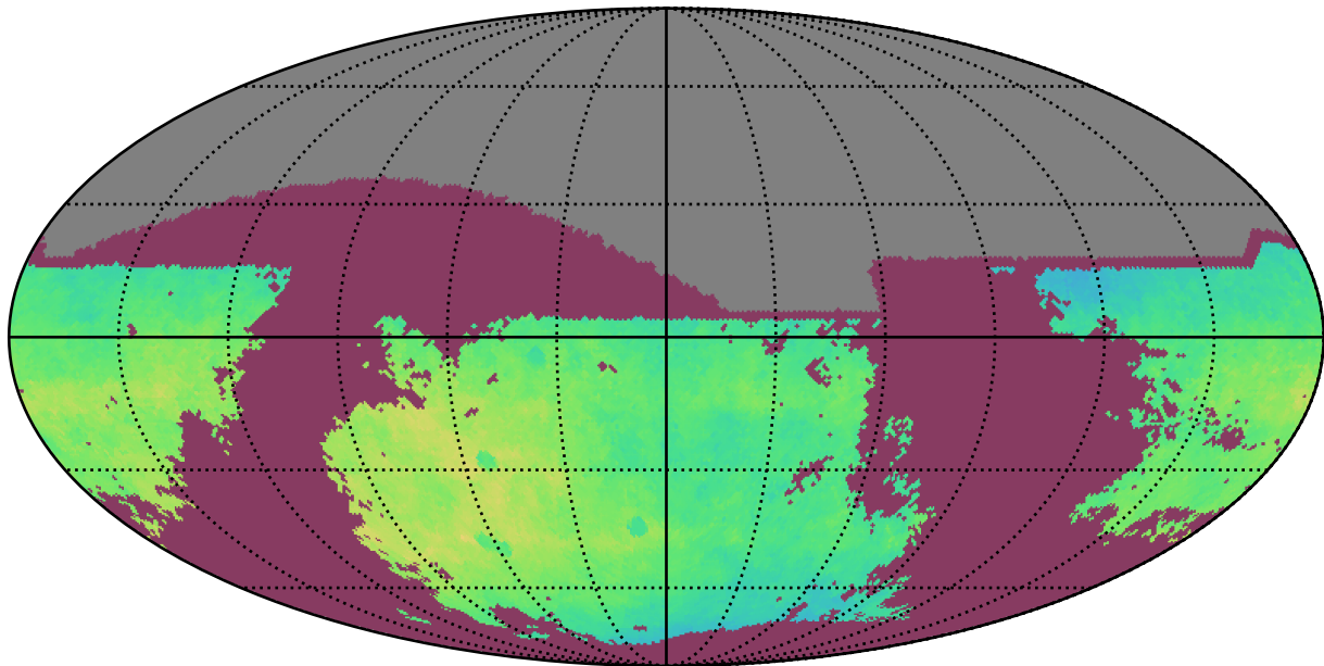
too_combined_no_nss_s10.0_v3.4_10yrs i: NgalScale
