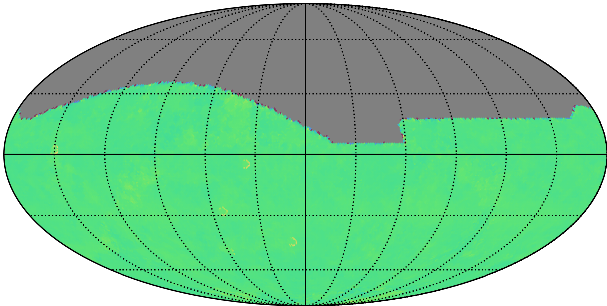
too_combined_no_nss_s10.0_v3.4_10yrs i: Kuiper rotTelPos
