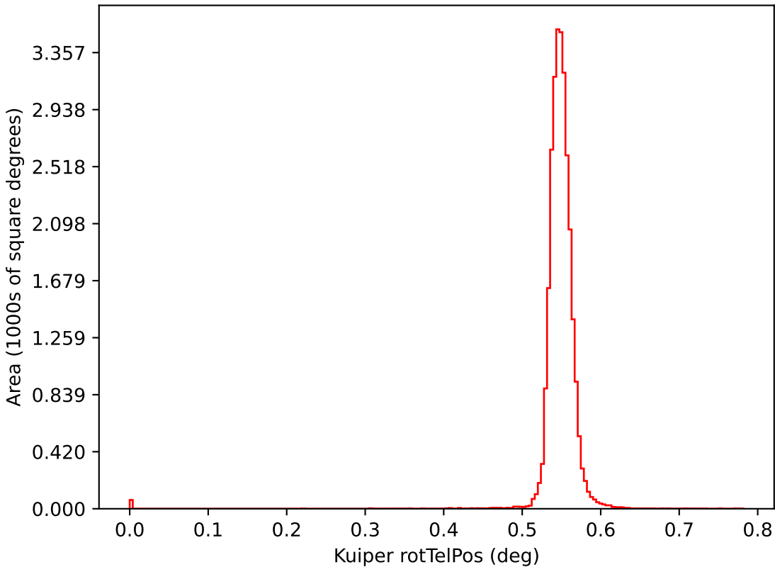
too_combined_no_nss_s10.0_v3.4_10yrs i: Kuiper rotTelPos
