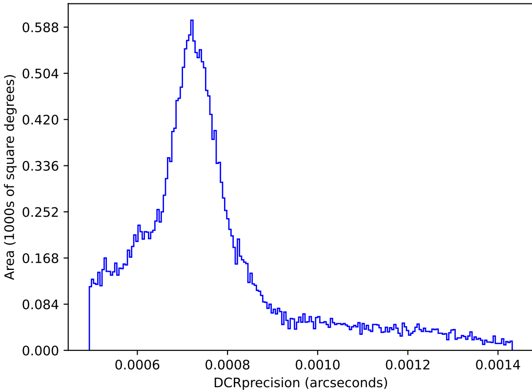
too_combined_no_nss_s10.0_v3.4_10yrs : DCRprecision
