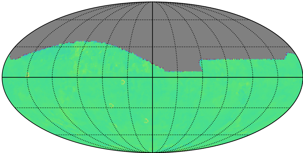
too_combined_no_gw_s10.0_v3.4_10yrs z: Kuiper rotTelPos
