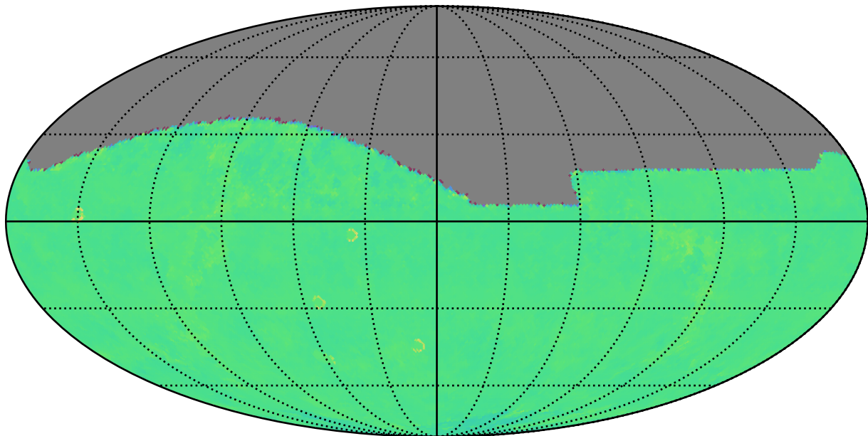
too_5_4v3.4_10yrs z: Kuiper rotTelPos
