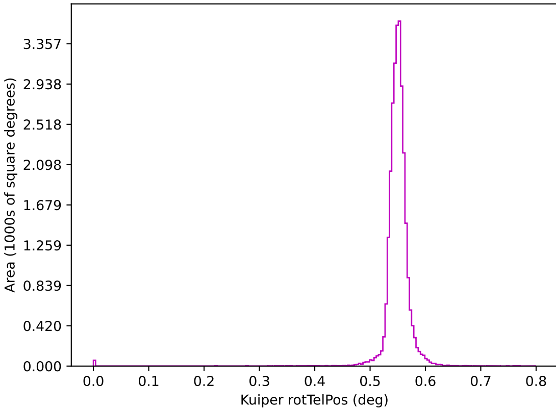
too_5_4v3.4_10yrs z: Kuiper rotTelPos
