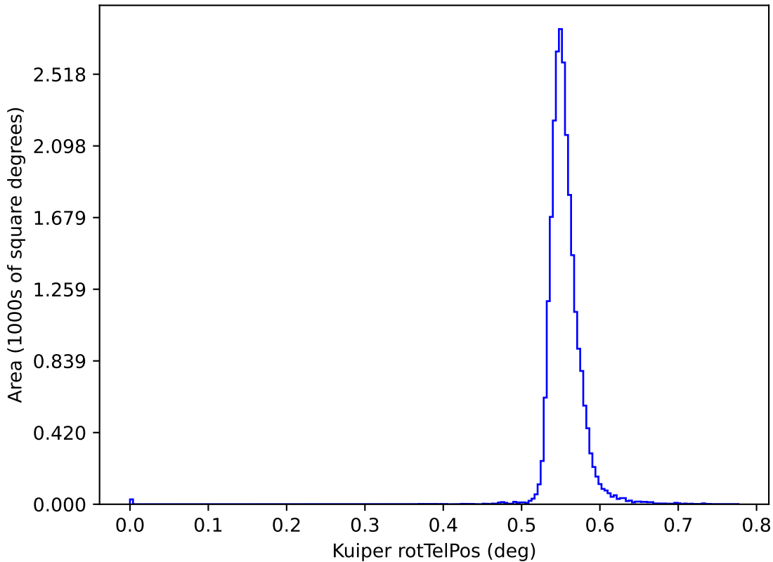
too_5_4v3.4_10yrs y: Kuiper rotTelPos
