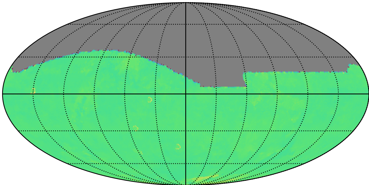
too_5_4v3.4_10yrs r: Kuiper rotTelPos
