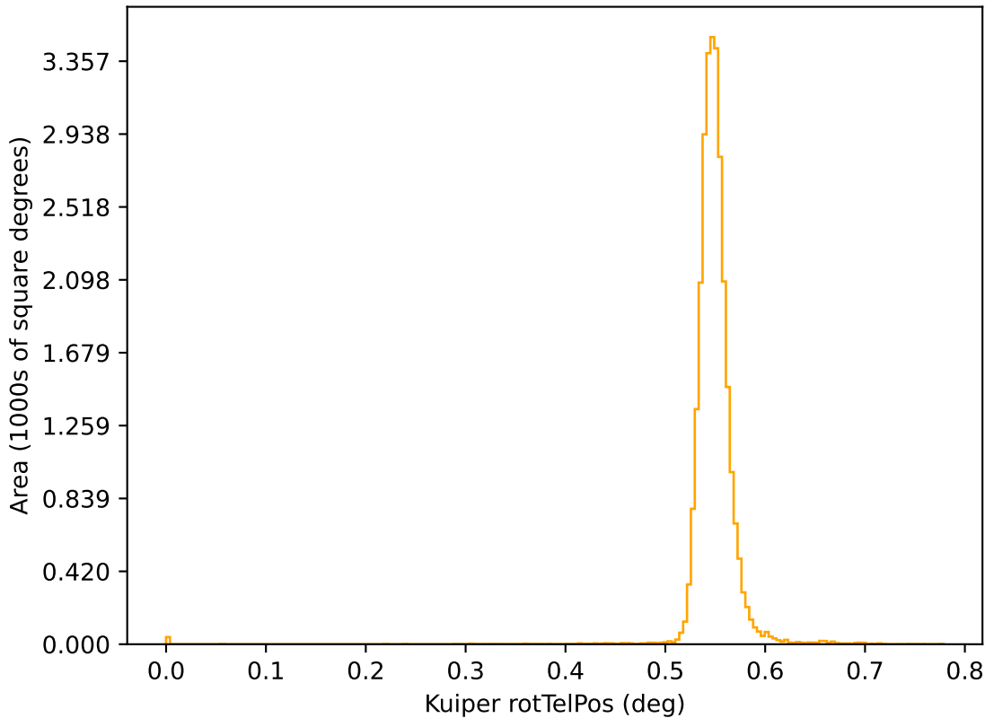
too_5_4v3.4_10yrs r: Kuiper rotTelPos
