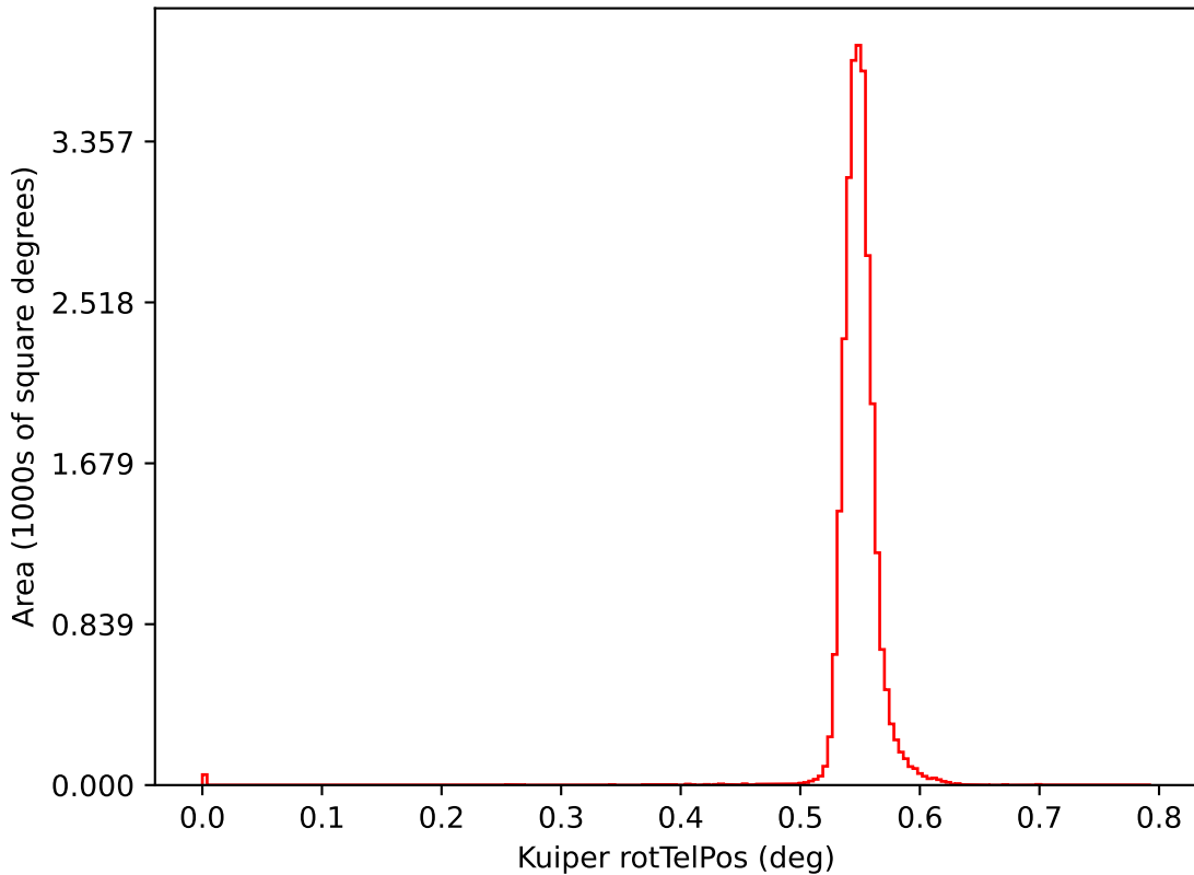
too_5_4v3.4_10yrs i: Kuiper rotTelPos
