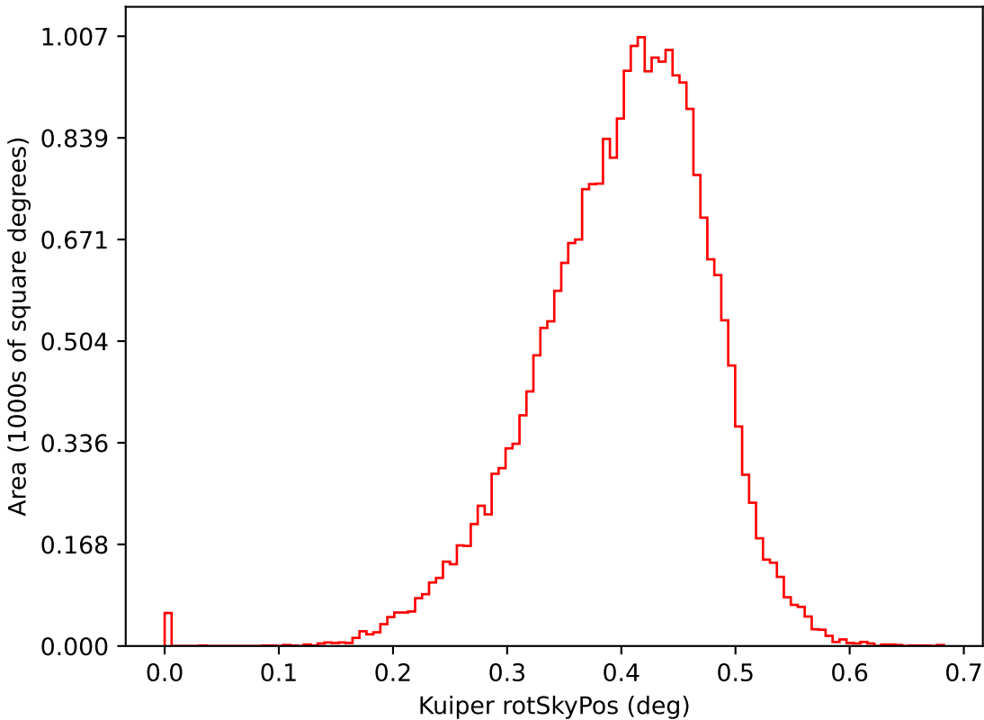
too_5_4v3.4_10yrs i: Kuiper rotSkyPos
