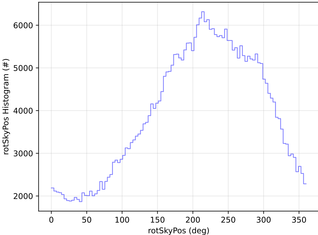
too_5_4v3.4_10yrs All sky y band: rotSkyPos Histogram
