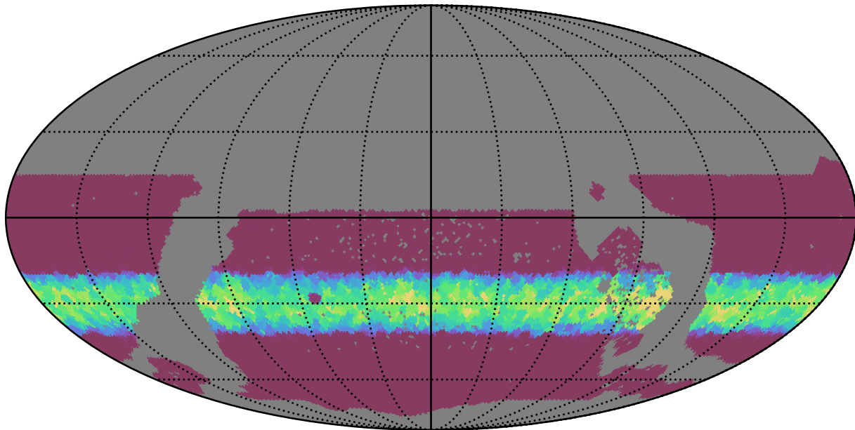
too_5_4v3.4_10yrs WFD y band: Min normairmass
