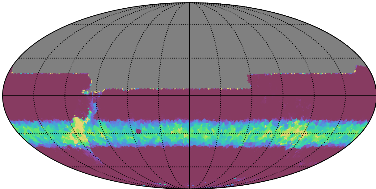
too_5_4v3.4_10yrs All sky y band: Min normairmass
