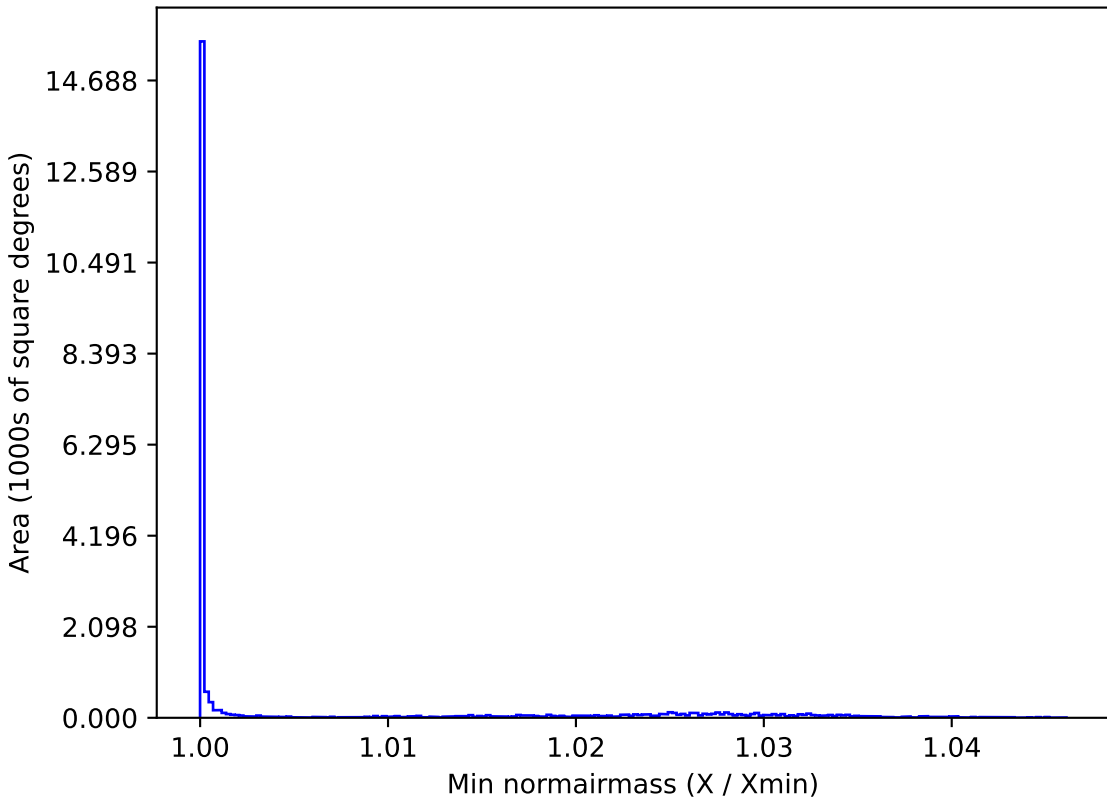
too_5_4v3.4_10yrs All sky y band: Min normairmass
