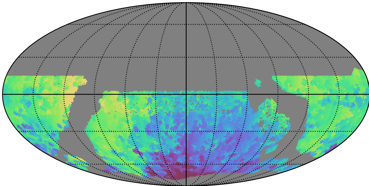
too_5_4v3.4_10yrs WFD y band: Min HA
