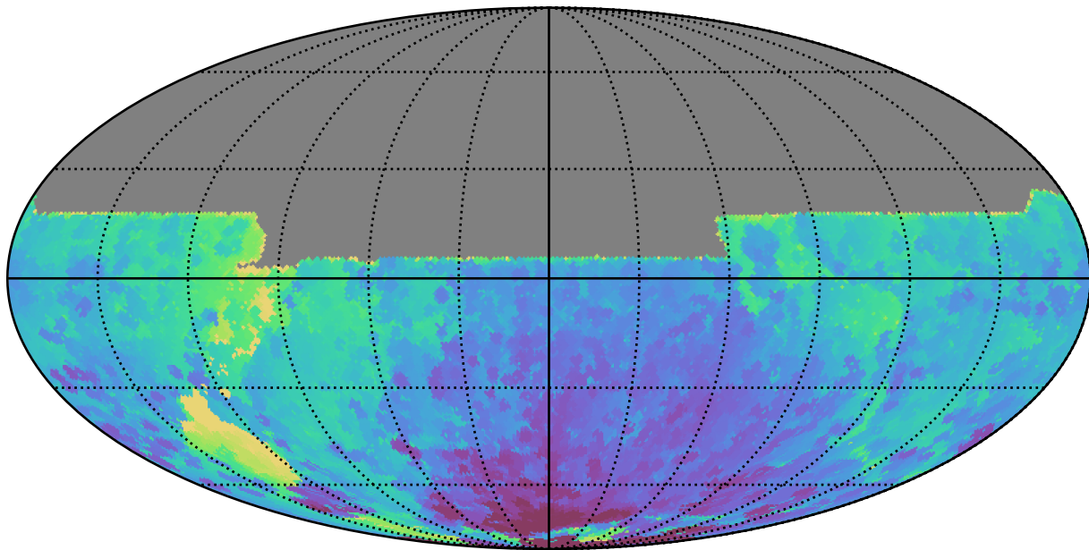
too_5_4v3.4_10yrs All sky y band: Min HA
