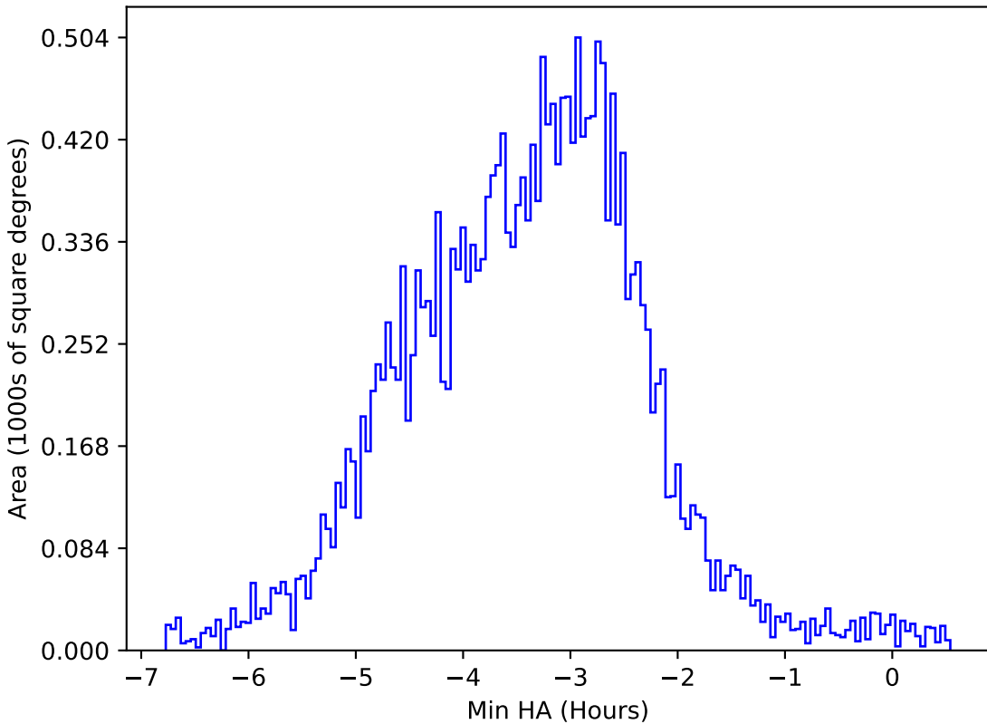
too_5_4v3.4_10yrs All sky y band: Min HA
