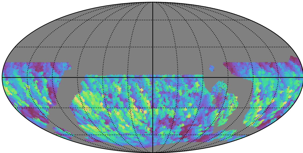
too_5_4v3.4_10yrs WFD y band: Max normairmass
