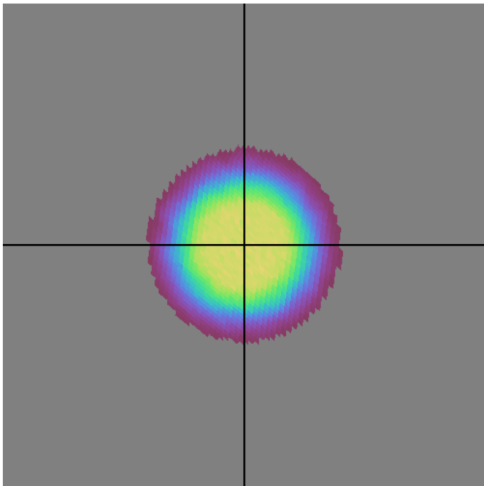
too_5_4v3.4_10yrs r band: DD:ELAISS1 NVisits
