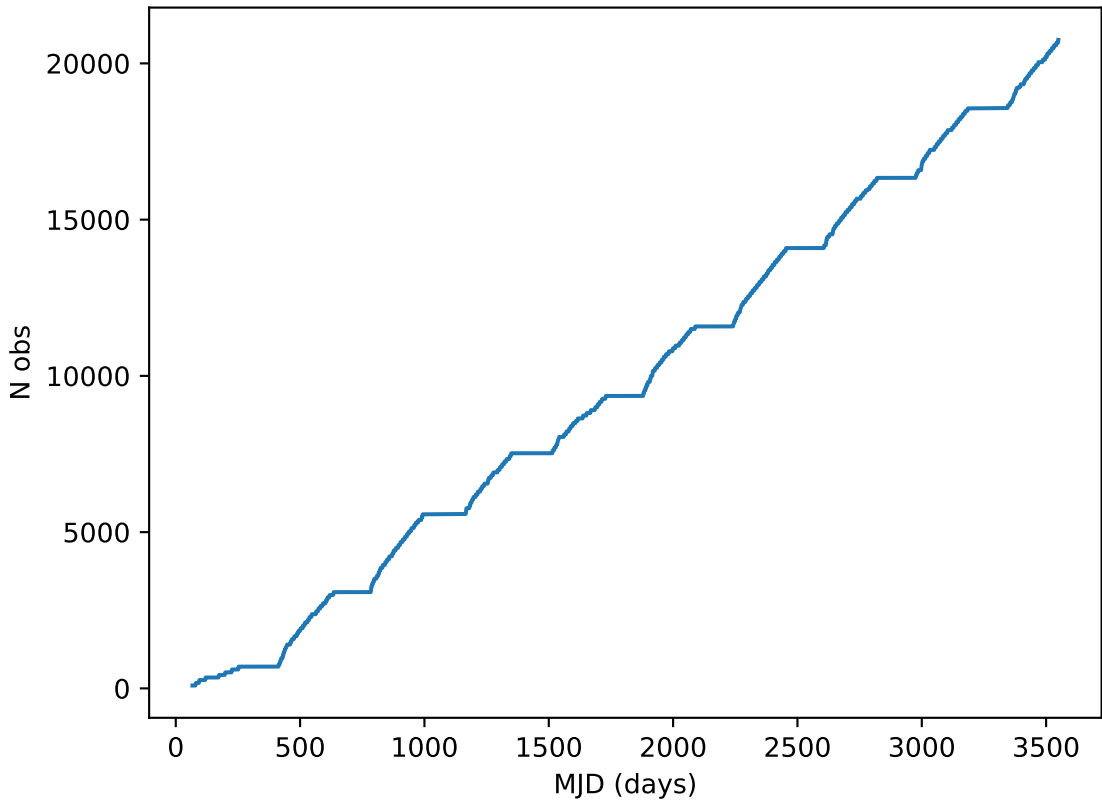
too_5_4v3.4_10yrs all bands: DD:ELAISS1 Cumulative NVisits
