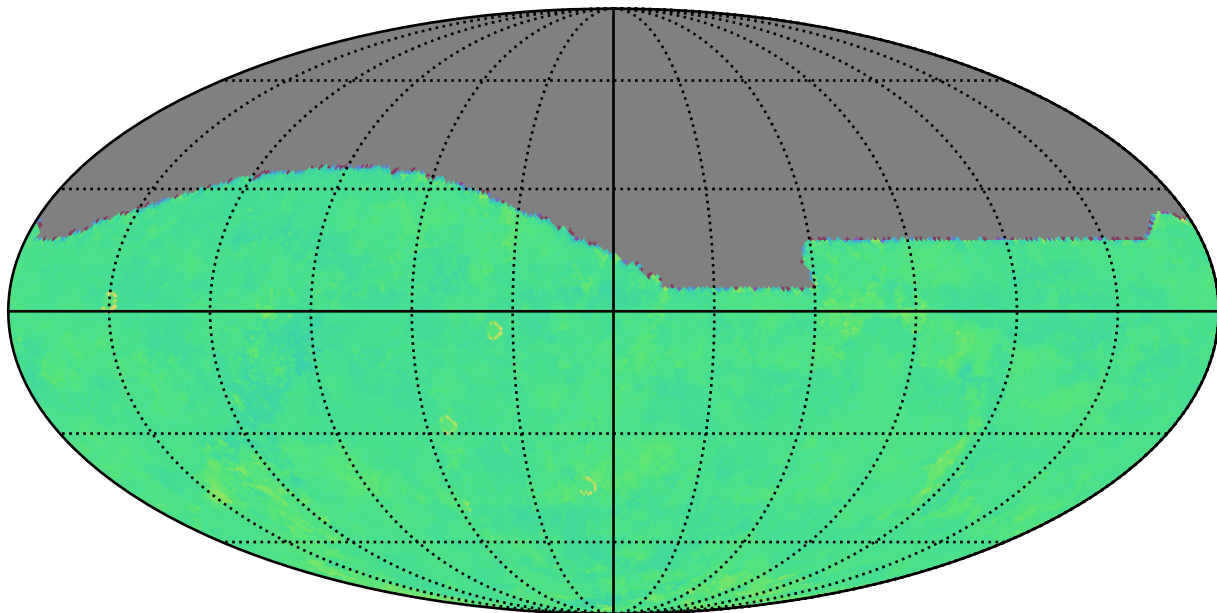
too_5_1v3.4_10yrs g: Kuiper rotTelPos
