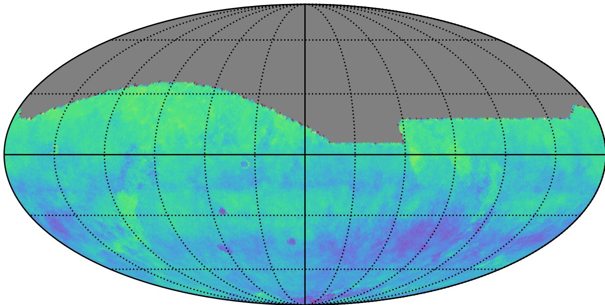
too_5_1v3.4_10yrs i: Kuiper rotSkyPos
