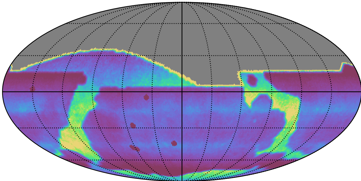
too_5_1v3.4_10yrs : DCRprecision
