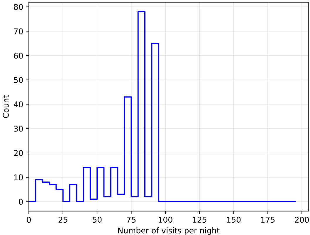
too_5_1v3.4_10yrs all bands: DD:ELAISS1 NVisitsPerNight
